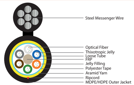
48 Fiber 6x8
