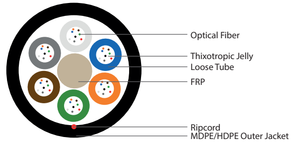
48 Fiber 6x8
