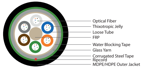
48 Fiber 6x8
