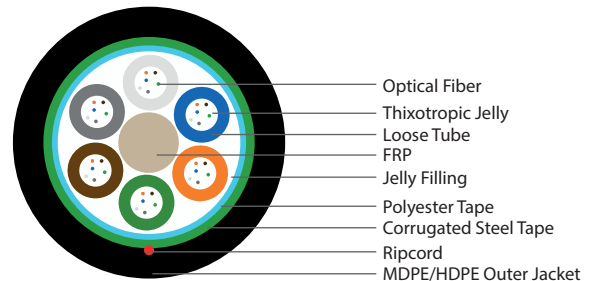
48 Fiber 6x8
