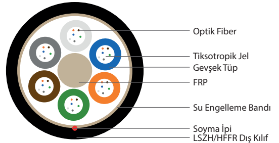
48 Fiber 6x8
