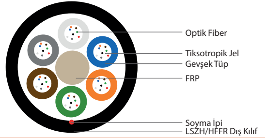
48 Fiber 6x8
