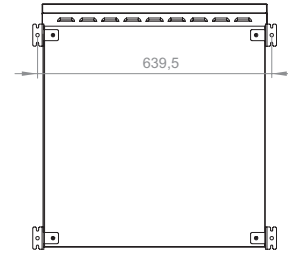
Arka görünüş
