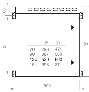
Ön görünüş
